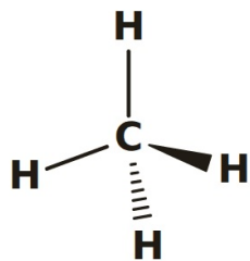
CH 4 : 109.5° 4 bonding pairs, 0 lone pairs
