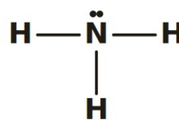
NH 3 : 4 domains 3 bonds + 1 lone pair
